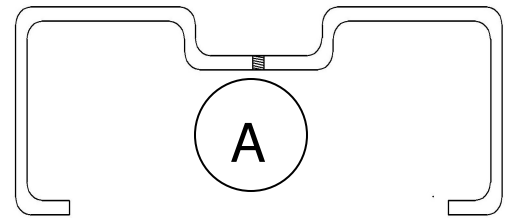
Strike Jamb (x1)
